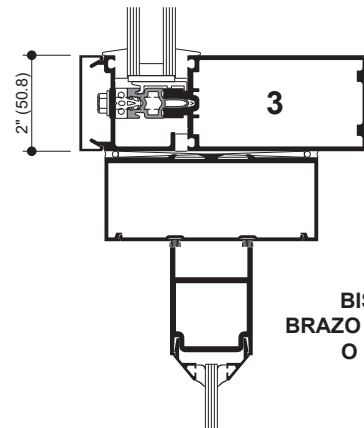
DINTEL BISAGRA PLANA O BISAGRA DE PIVOTE CON BRAZO DE CIERRE SUPERIOR OCULTO DE ACCIÓN SENCILLA
