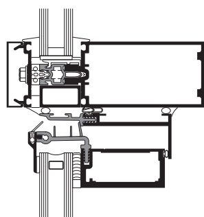
CABEZAL
