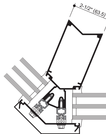
ESQUINA EXTERIOR DE 135°
