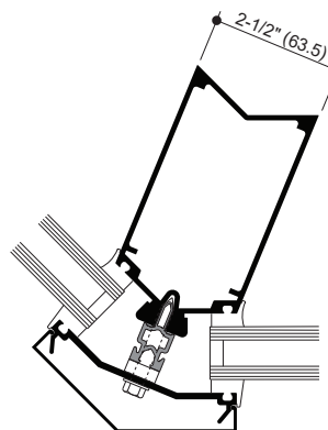
ESQUINA EXTERIOR DE 135°
