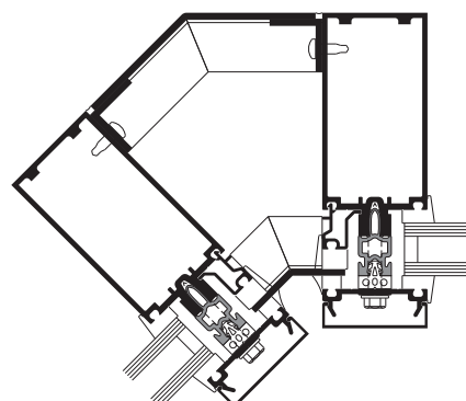
ESQUINA INTERIOR DE 135°
