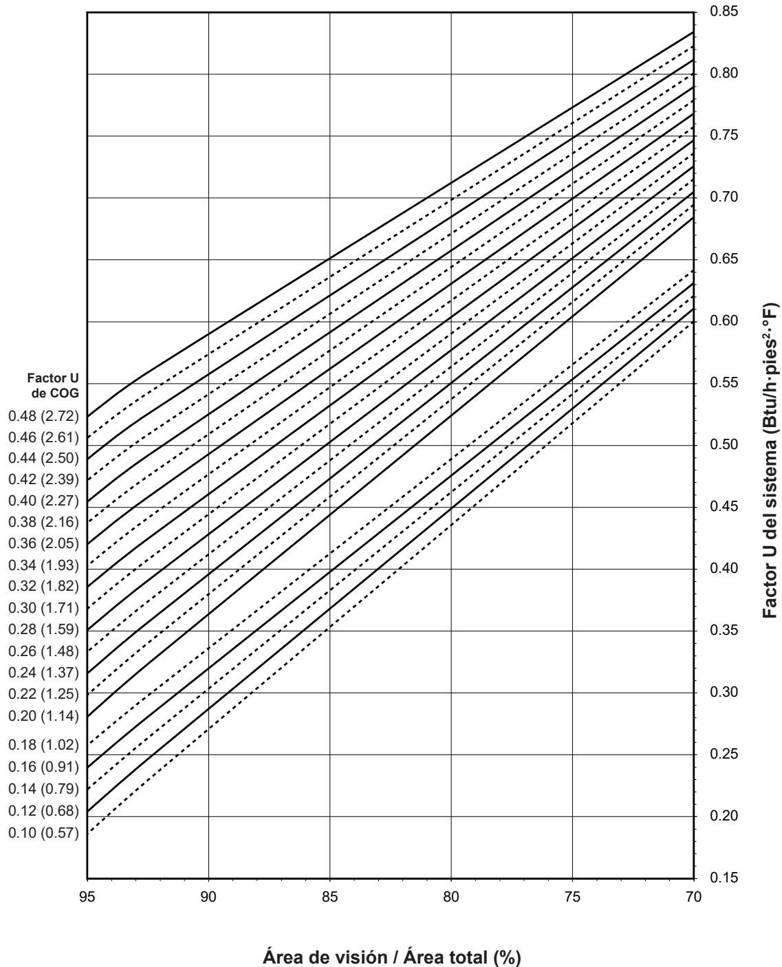
Factor U del sistema para el vidrio de visión
