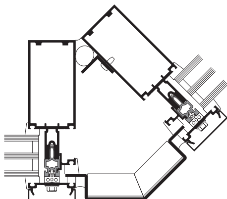
ESQUINA EXTERIOR DE 135°
