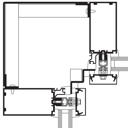
ESQUINA INTERIOR DE 90°
