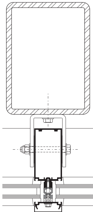
ANCLAJE A ACERO ESTRUCTURAL VERTICAL
