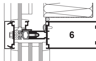
TRAVESAÑO - ANTEPECHO SOBRE VISIÓN
