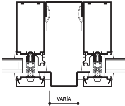
MONTANTE DOBLE
