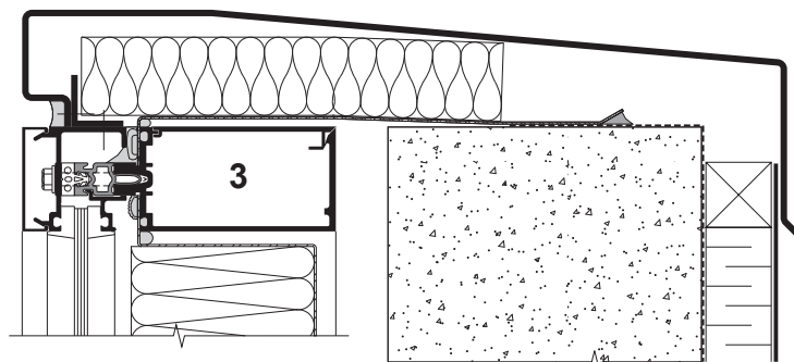
TRAVESAÑO SUPERIOR A RAS DEL PARAPETO
