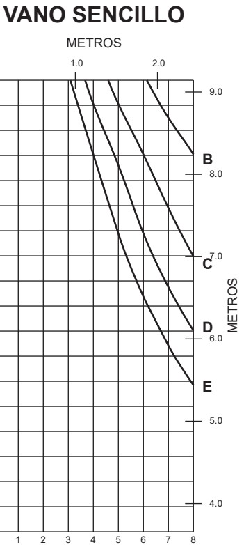
CENTROS DE MONTANTES EN PIES
