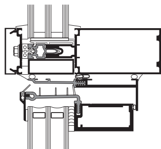
CABEZAL
