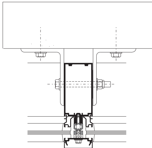
ANCLAJE A ACERO DE SOPORTE
