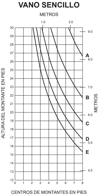
CENTROS DE MONTANTES EN PIES
