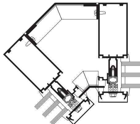
ESQUINA INTERIOR DE 135°
